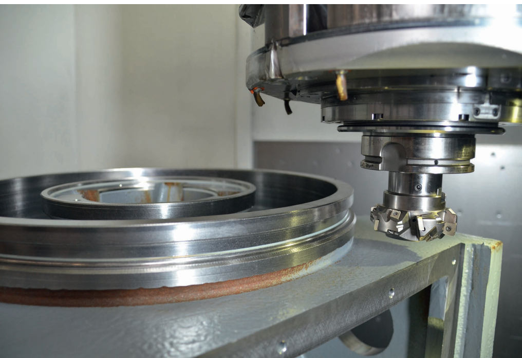
1 Der ultra-kompakte Sonderfräser, den Avantec für Expert-Tünkers entwickelte, nach dem Schruppfräsen des Kugelkranzes an einem Drehtisch-Gehäuse (© Hanser)
